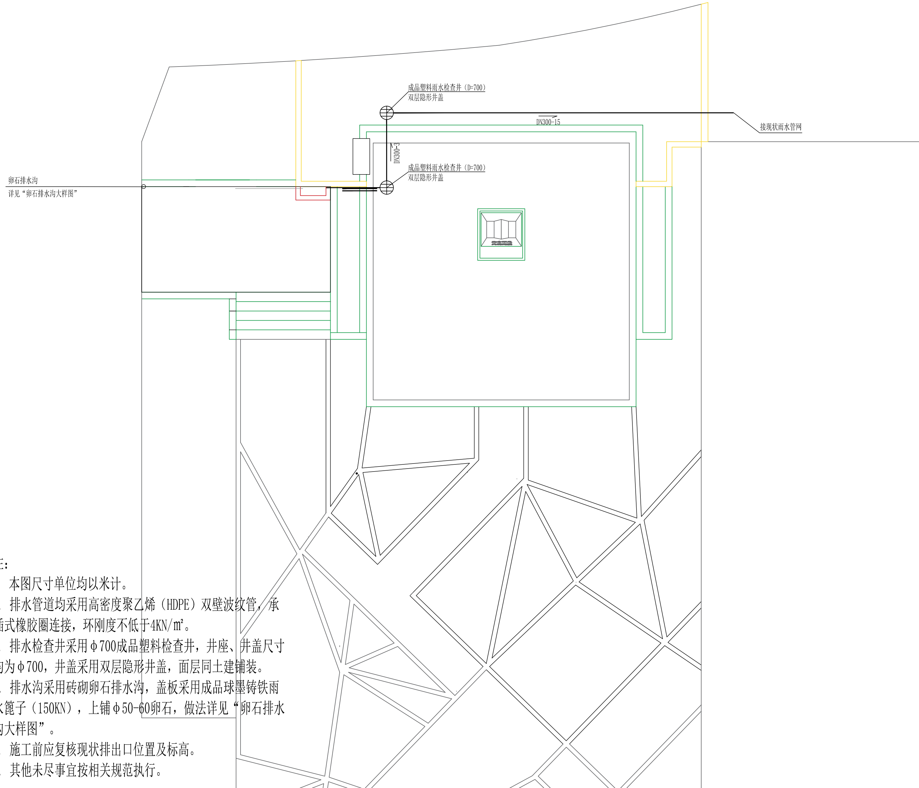
排水平面图 1:100
